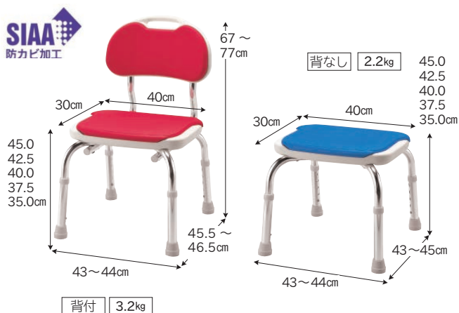
シャワーベンチCPE-N 介・購入 S0300 背付 レッド 536-302 ブルー 536-300 各¥18,150(税込) 背なし レッド 536-312 ブルー 536-310 各¥13,750(税込) 座面高さ 5段階調整、耐荷重 100kg アロン化成㈱
