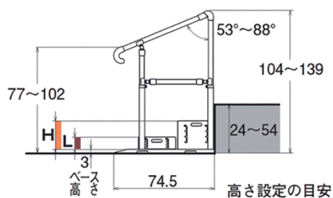
CKH-02 設置例
